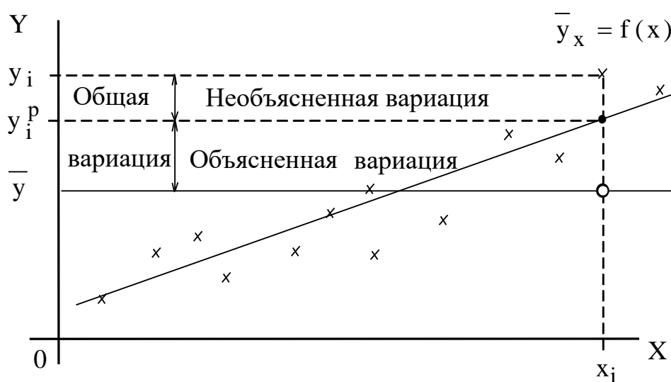
Рисунок 7 - Графическая интерпретация коэффициента детерминации для случая линейной регрессии
