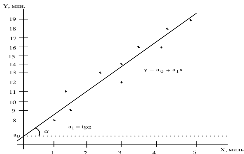
Рисунок 8 - График исходных данных и предполагаемая линия регрессии
