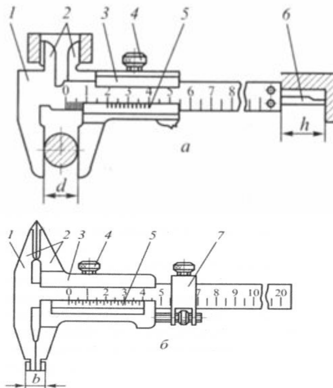
а- штангенциркуля ШЦ-1
