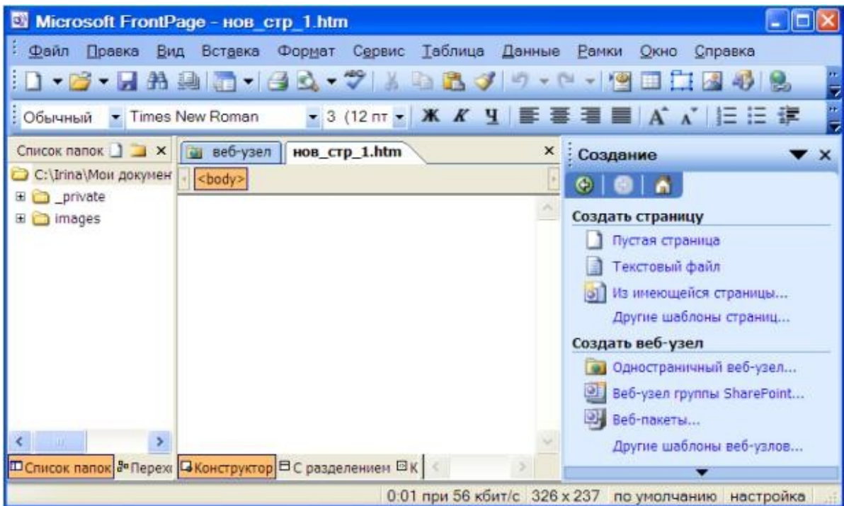
Рисунок 12 - Окно FrontPage
