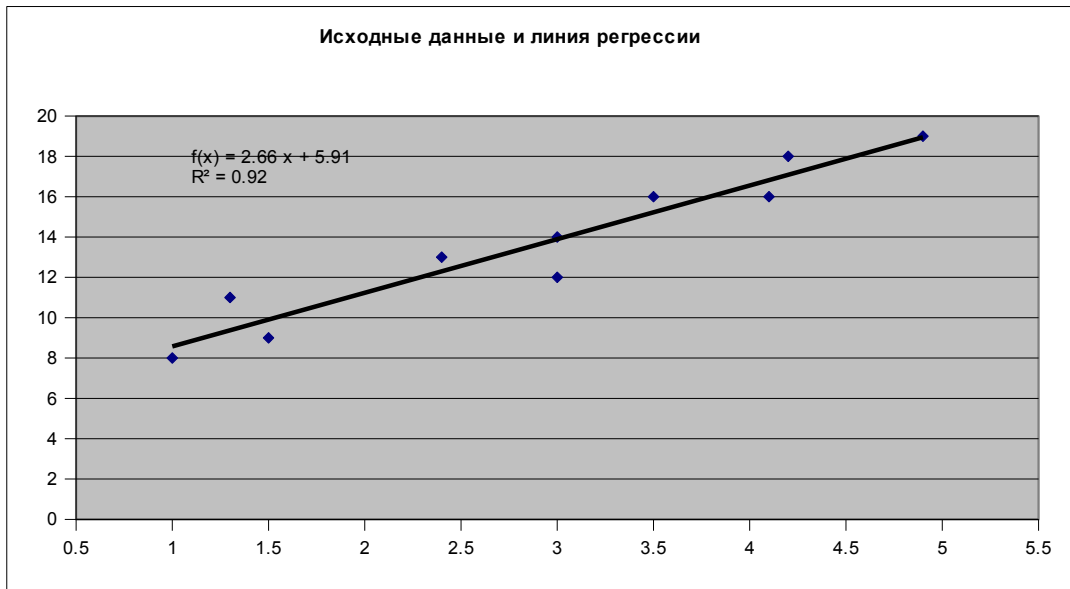
Рисунок 10 - Линия регрессии
