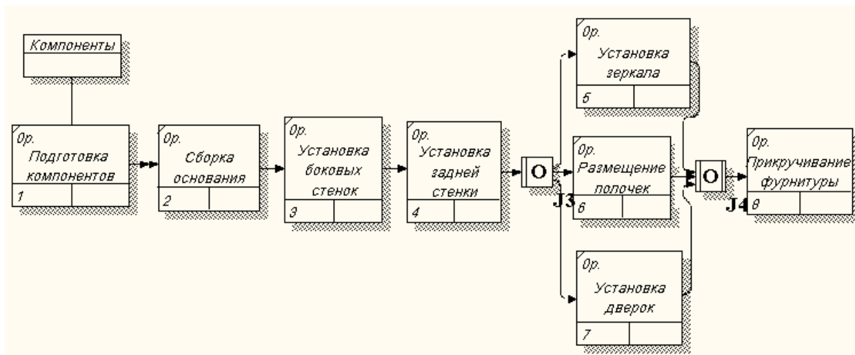
Рисунок 92 - Диаграмма IDEF3
