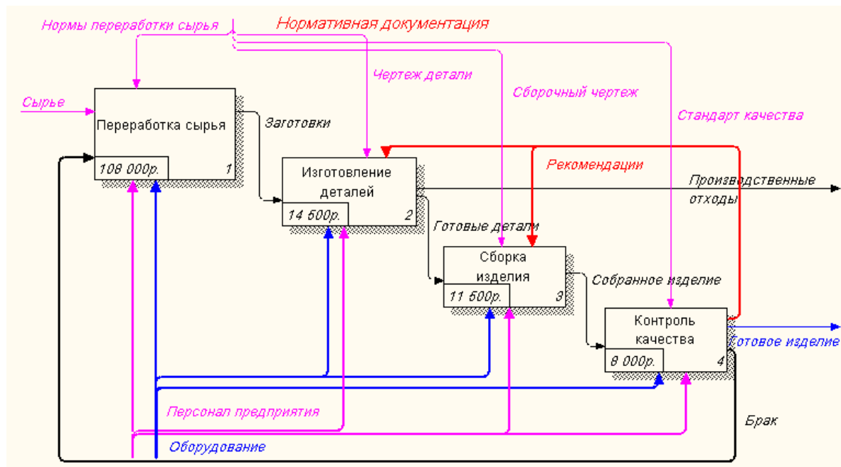
Рисунок 101 - Результат стоимости работ на диаграмме A1
