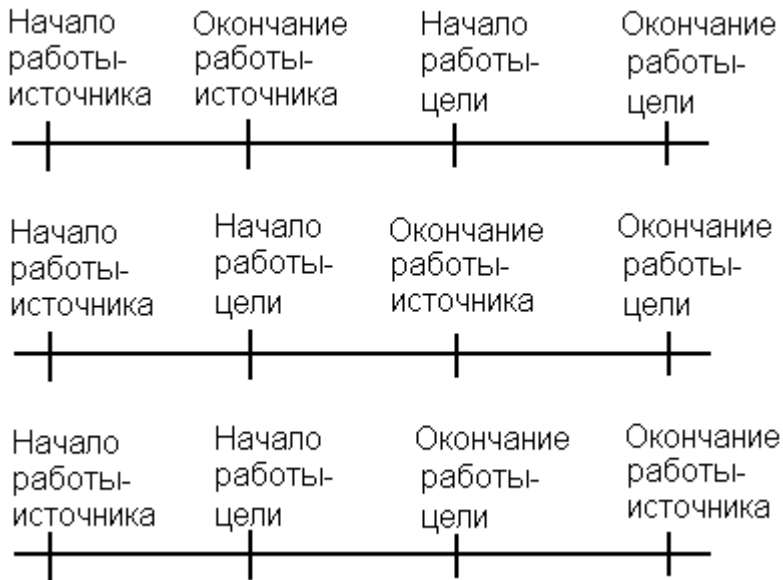
Рисунок 78 - Временная диаграмма выполнения работ
