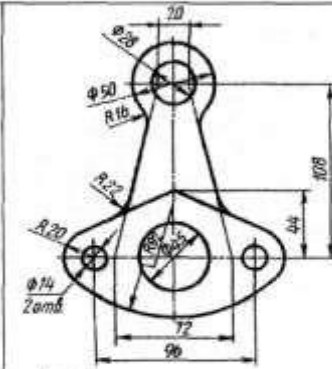
Рычаг
