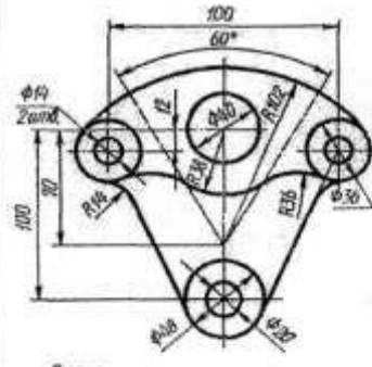
Вилка
