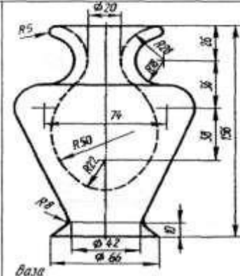
База
