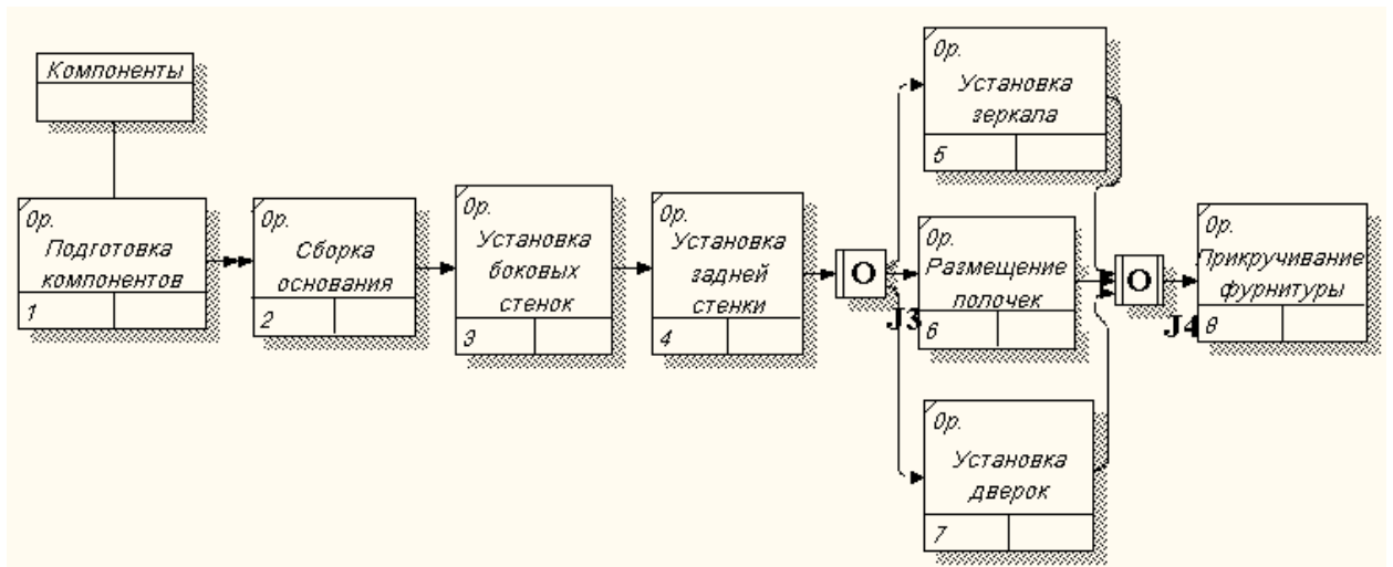
Рисунок 92 - Диаграмма IDEF3
