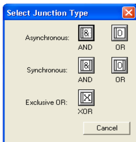
Рисунок 79 - Типы перекрестков
