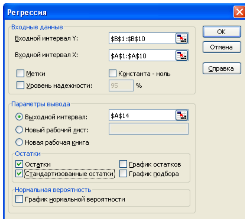
Рисунок 9 – Окно Регрессия
