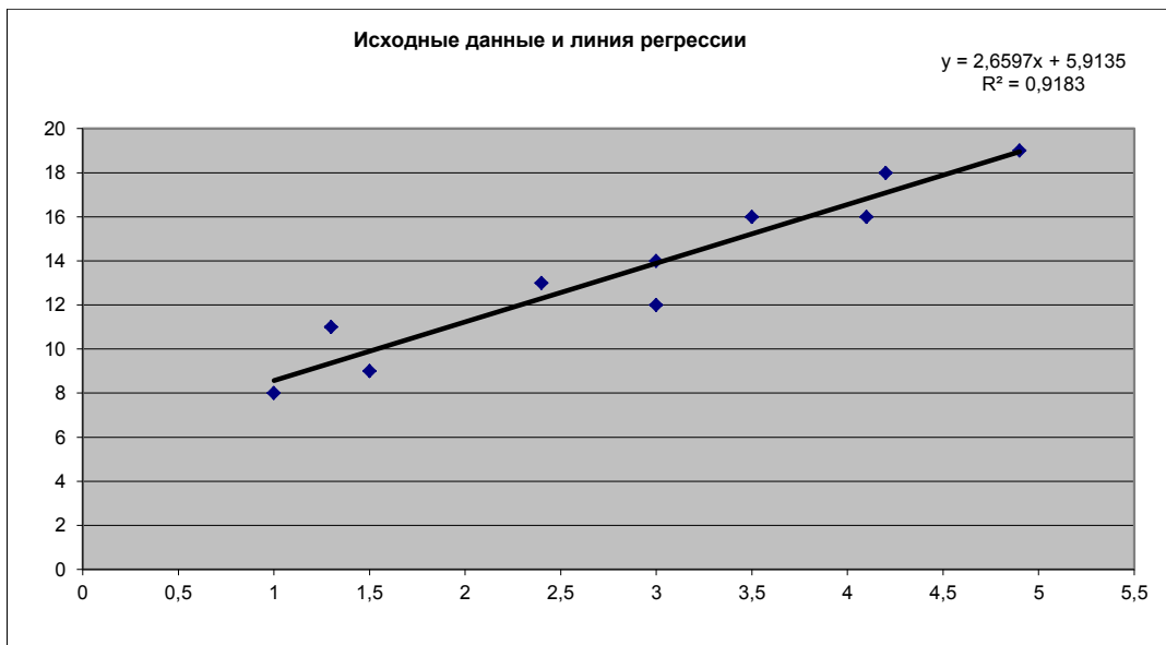
Рисунок 10 - Линия регрессии
