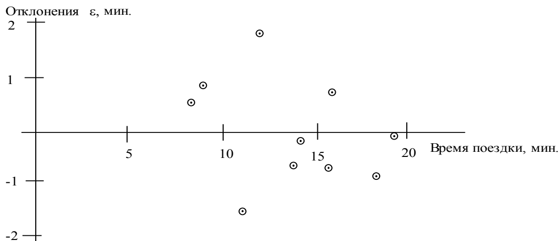
Рисунок 11 - График отклонений
