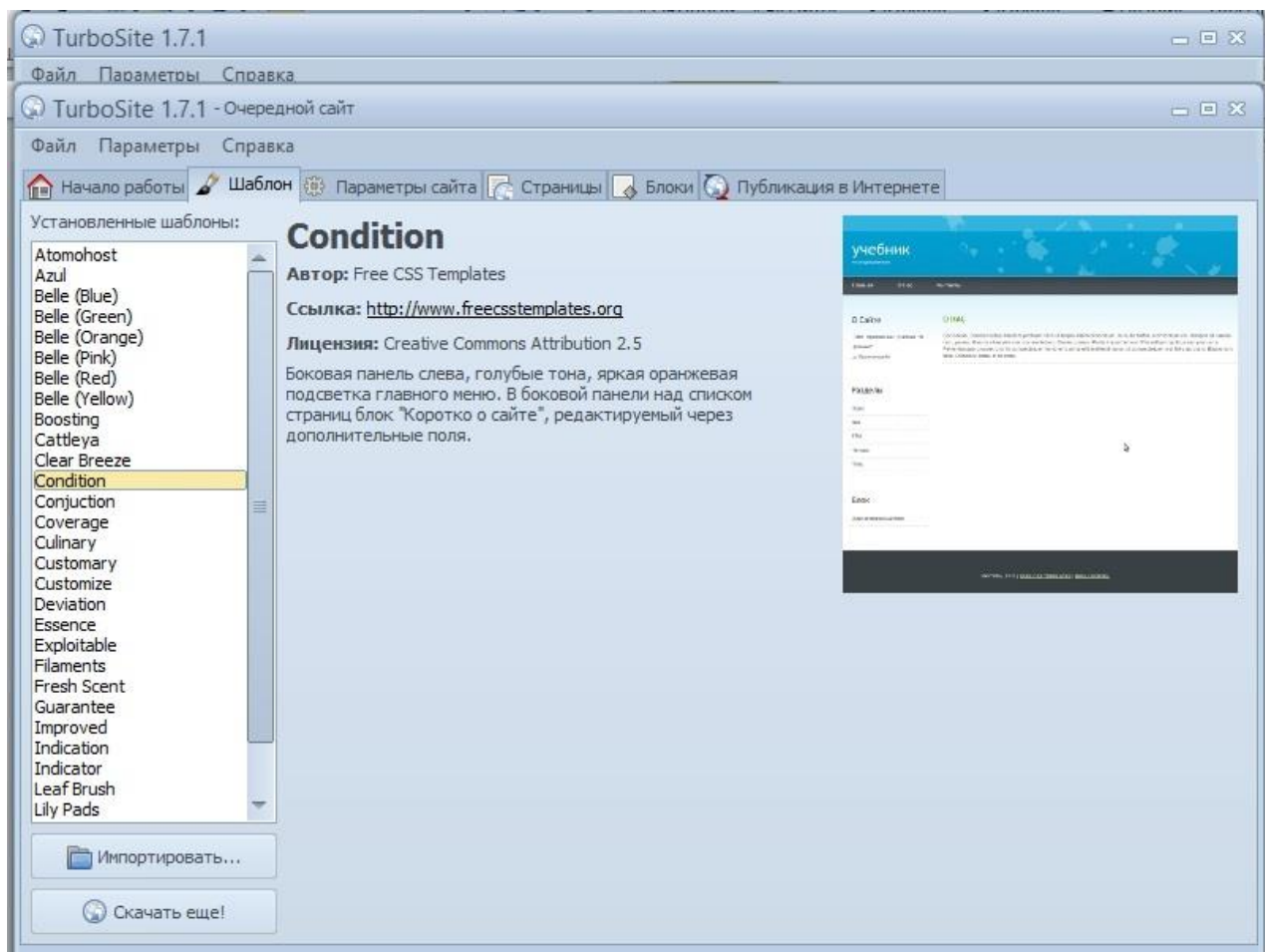
Рисунок 26 – Вкладка Шаблон
