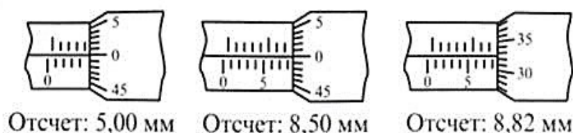
Рисунок 2.6 – Шкалы микрометра
