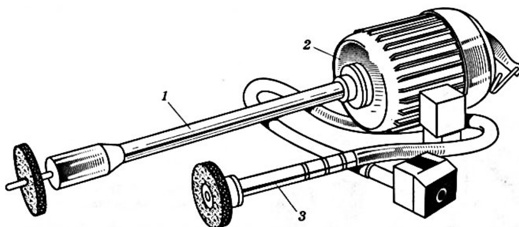
Рисунок 3.9 – Шероховальный станок с гибким приводом и сменными валами: 1 – жесткий вал с цилиндрической проволочной щеткой; 2 - электродвигатель; 3 – гибкий вал
