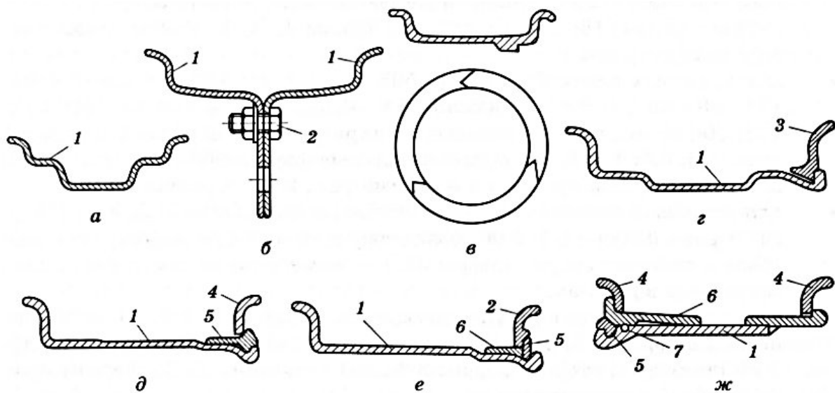
Рисунок 1.8. Основные типы ободьев колес:
