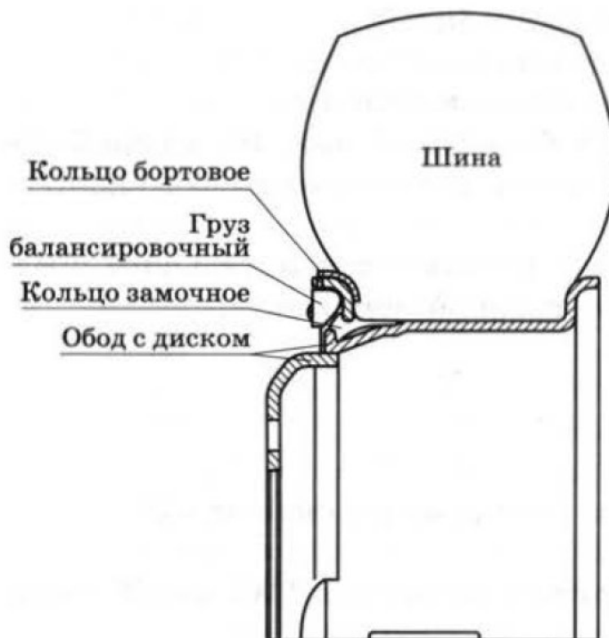
Рисунок 1.6 – Дисковое колесо
