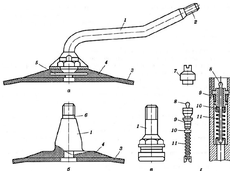
Рисунок 1.5 - Вентили
