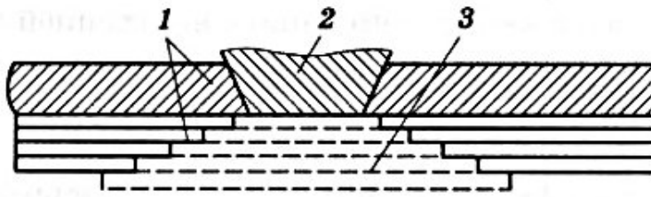
Рисунок 3.16 – Заделка повреждения в случае вырезания участка способом «в рамку»: 1 – прослоечная резина; 2 – протекторная резина; 3 – слой корда
