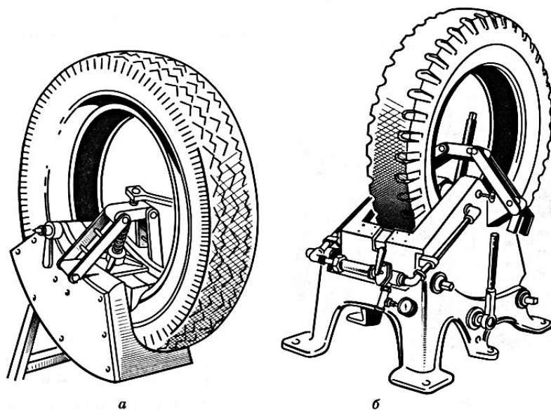
Рисунок 3.20 – Мულды для ремонта покрышек: а – специализированная; б - универсальная
