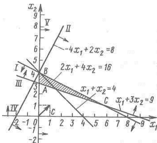
Рисунок 2.1 - Графическая интерпретация решения задачи линейного программирования 1
