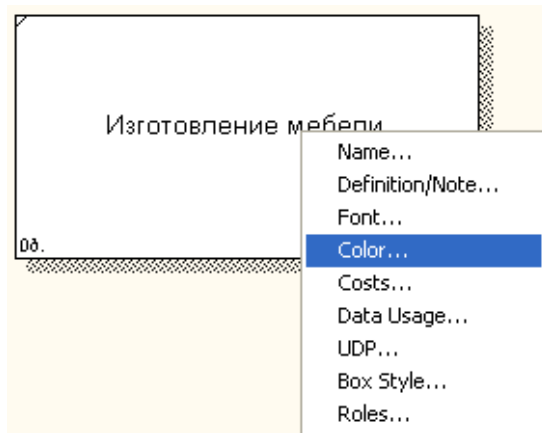
Рисунок 25 Контекстно-зависимое меню
