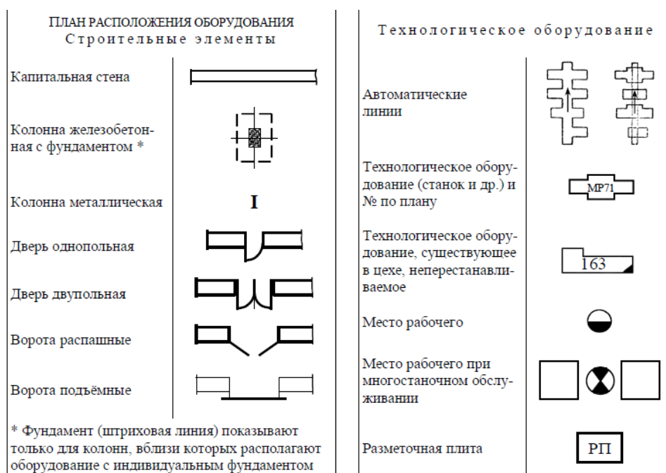
Рисунок 6.1 - План расположения строительных элементов и технологического оборудования.
