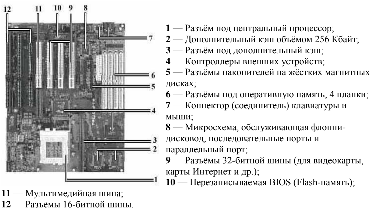
Рис. 2.9. Системная плата компьютера класса Pentium
