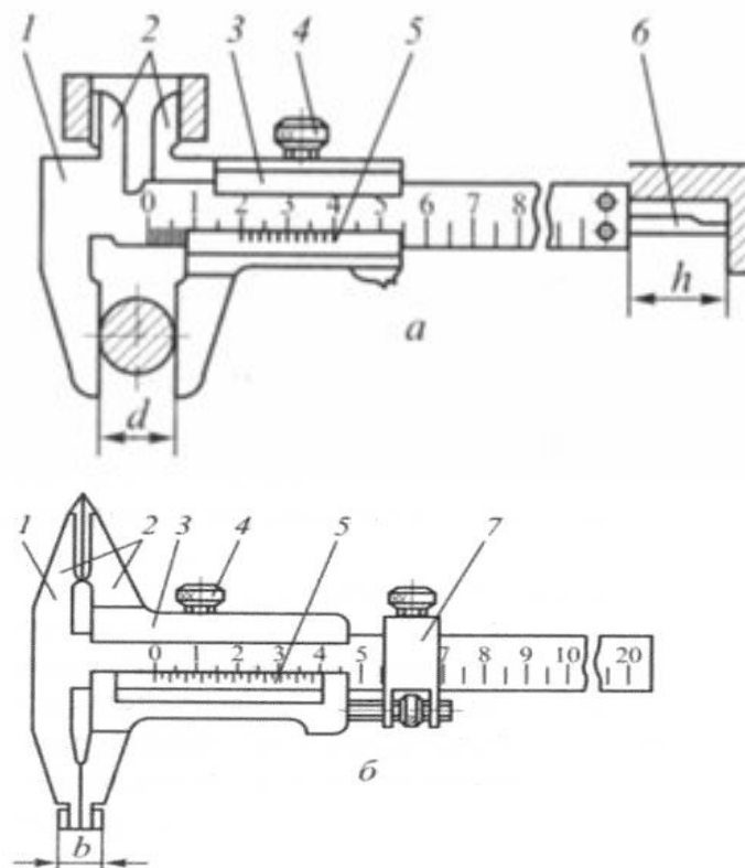
а- штангенциркуль ШЦ-1
