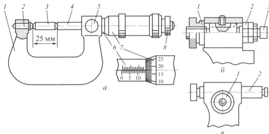
а – устройство: 1 – скоба; 2 – пятка; 3 – установочная мера; 4 – микровинт; 5 – стопор; 6 – стебель; 7 – барабан; 8 – трещотка; б – сменная пятка: 1, 2 – гайка; 3 – пятка; в – регулируемая пятка: 1 – фиксатор; 2 – пятка.
