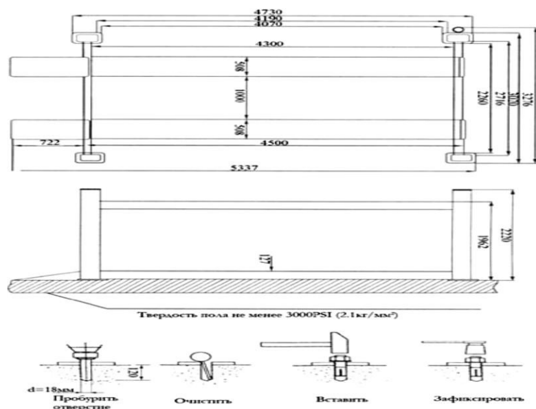
Рисунок 3.1 – Общий вид подъёмника
