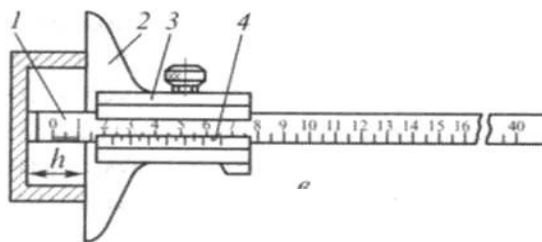
Рисунок 2.2 – Штангенглубиномер
