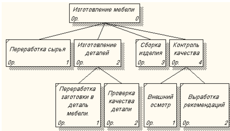
Рисунок 59 - Дерево узлов
