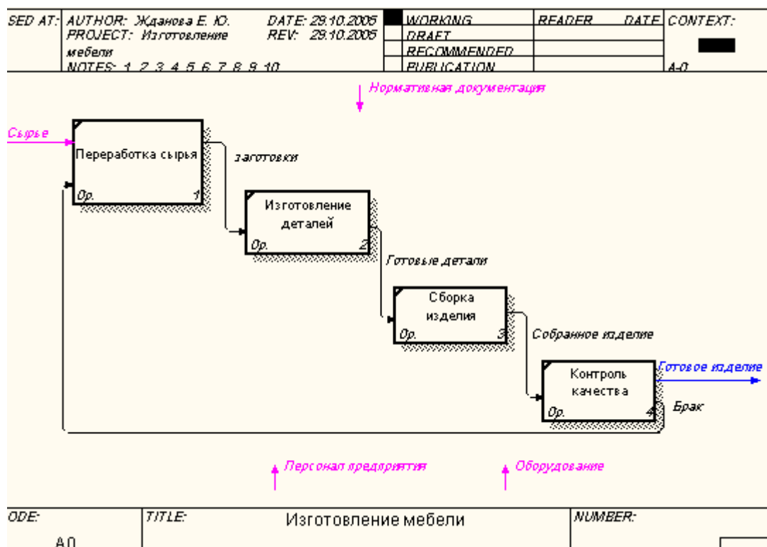
Рисунок 36 - Процесс декомпозиции
