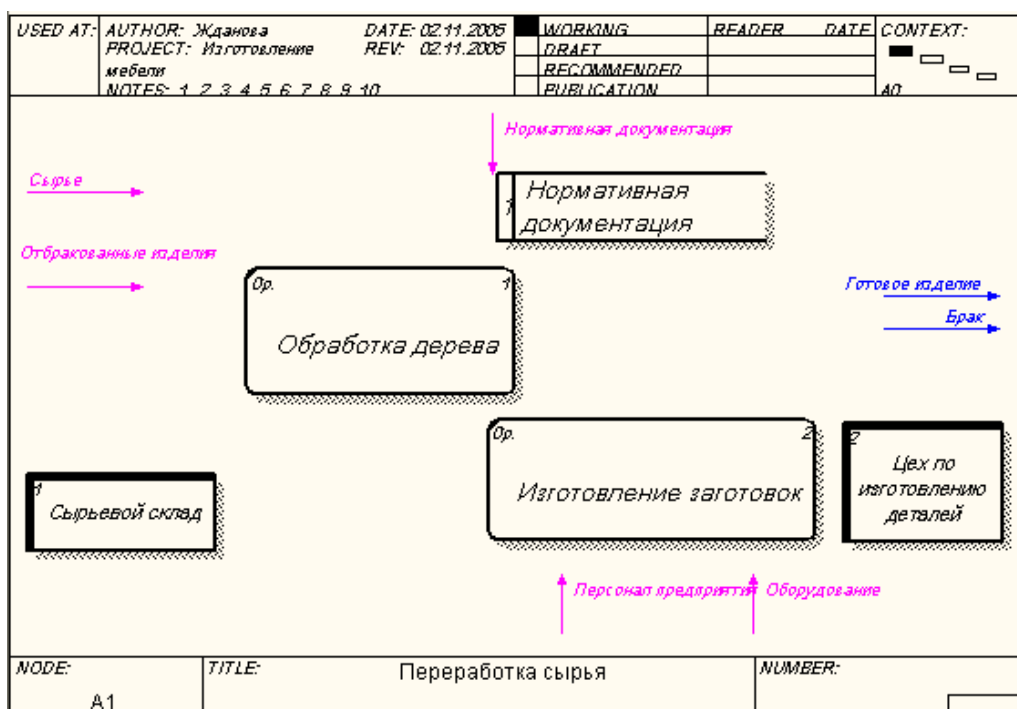
Рисунок 73 - Диаграмма DFD
