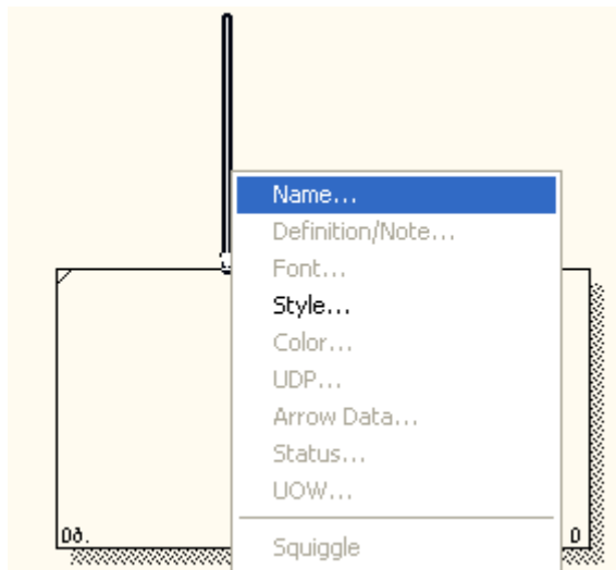
Рисунок 17 - Контекстно-зависимое меню
