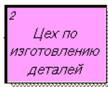
Рисунок 66 - Внешняя сущность
