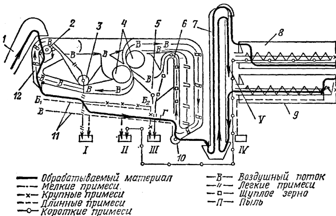
Рис.26. Функциональная схема сеяноочистительной машины СМ-4: 1 - загрузочный транспортер; 2 — распределительный шнек; 3 — шнек отходов; 4- роторы вентиляторов; 5 — отстойная камера; 6 - рабочий канал второй аспирации; 7 — двухпоточный элеватор; 8 — триерный цилиндр для выделения коротких примесей; 9 - триерный цилиндр для выделения длинных примесей; 10 — шнек очищенного зерна; 11 - решетный стан; 12 — рабочий канал первой аспирации; I — выход легких и мелких примесей; II — мелкое зерно и короткие примеси; III - крупные примеси и щуплое зерно; IV -длинные примеси; V-очищенное зерно.
