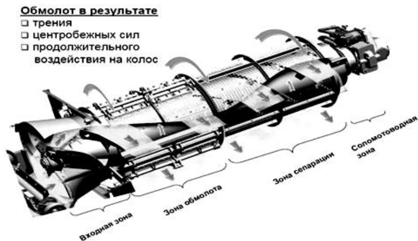
Рис.10. Молотильно-сепарирующее устройство роторного типа: вход – приемная часть ротора; обмолот – молотильная часть ротора; сепарация – сепарирующая часть ротора; выброс – выходное окно цилиндрического кожуха
