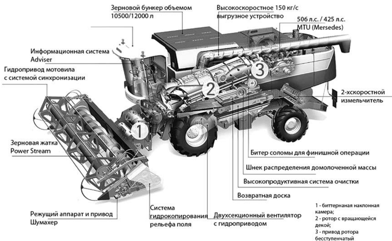
Рис. 9. Зерноуборочный комбайн РСМ-181 (Torum 750)
