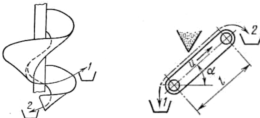
Рис.19. Схемы работы устройств, разделяющих материал по форме поверхности: винтовые сепараторы и продольные горки; 1 – выход округлых частиц; 2 – выход более плоских частиц
