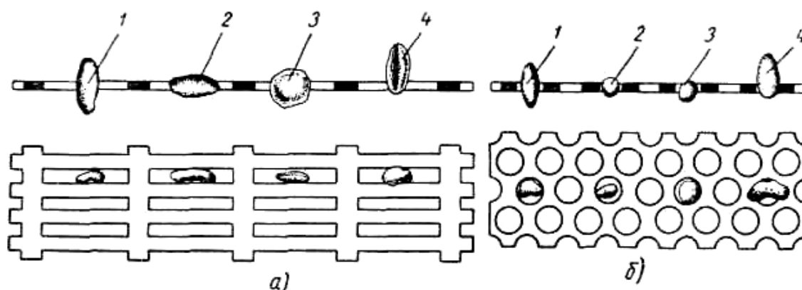
Рис.16. Разделение семян на решетках: а и б - разделение семян по толщине и ширине; 1, 2 и 3 – семя проходит сквозь отверстие; 4 – семя не проходит сквозь отверстие
