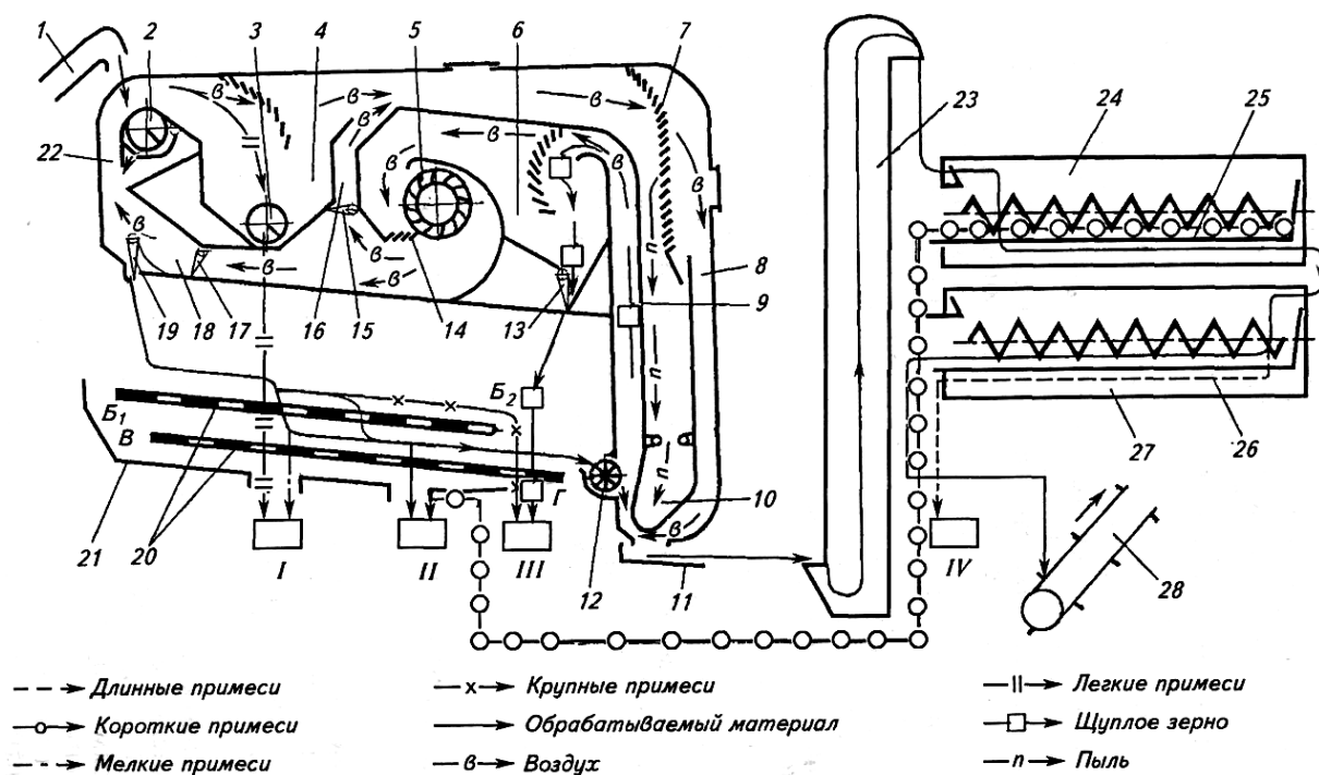
Рис.28. Функциональная схема семяочистительной машины МС – 4,5: 1,28 – соответственно загрузочный и отгрузочный транспортеры; 2,3 – шнеки; 4, 6 – соответственно, первая и вторая осадочные камеры; 5 – вентилятор; 7 – жалюзийный воздухоочиститель; 8, 18 – воздухоподводящие каналы; 9, 22 – соответственно второй и первый пневмосепарирующие каналы; 10 – пылесборник; 11 – вибродоток; 12 – питатель; 13, 19 – выпускные клапаны; 14 – жалюзийная перегородка; 15, 17 – регулировочные заслонки; 16 – перепускной канал; 20 – решетка; 21 – решетный стан; 23 – нория; 24, 27 – соответственно, кукольный и овсюжный цилиндрические триеры; 25, 26 – желоба
