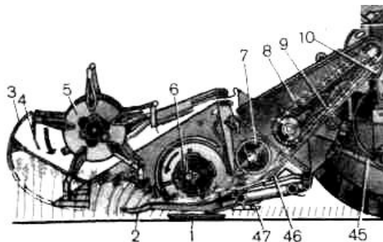
Рис.5. Схема технологического процесса работы жатвенной части комбайна «Енисей-1200М»: 1 – копирующий баашмак; 2 – режущий аппарат; 3 – делитель; 4 – граблина мотовила; 5 – мотовило; 6 – шнек жатки; 7 – битер проставки; 8 – наклонная камера; 9 – плавающий транспортер; 46 – проставка; 47 – рычаг
