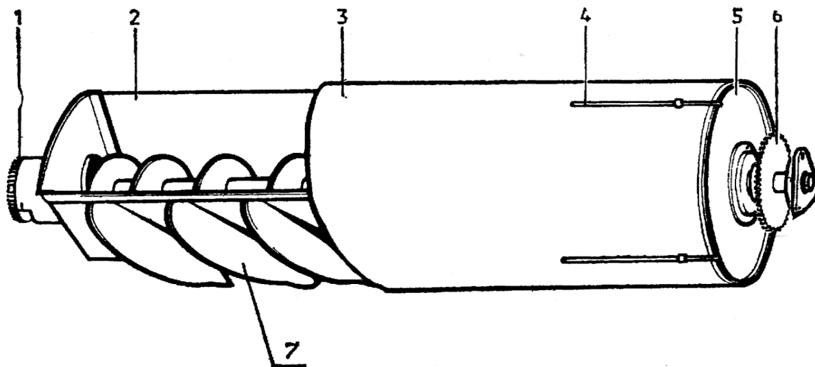
Рис.24. Триерный цилиндр: 1 - зубчатое колесо; 2 - лоток; 3 - обечайка; 4 - стяжка; 5 - розетка; 6 - приводная звездочка; 7 - плужок.
