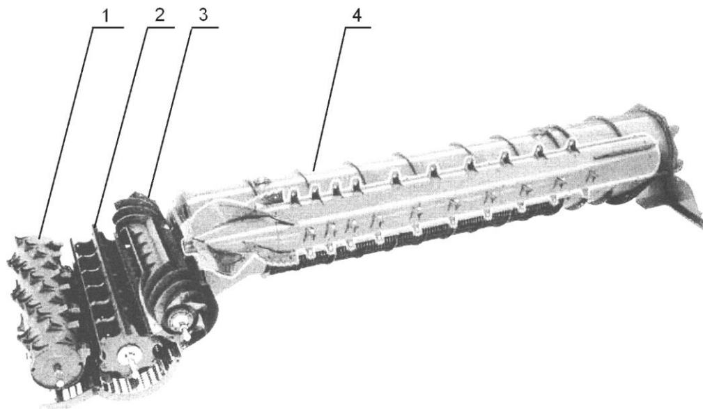
Рис.12. Система обмолота и сепарации комбайнов TUCANO 470/480: 1 – ускорительный барабан; 2 – обмолачивающий барабан; 3 – отбойный битер; 4 – роторный соломосепаратор
