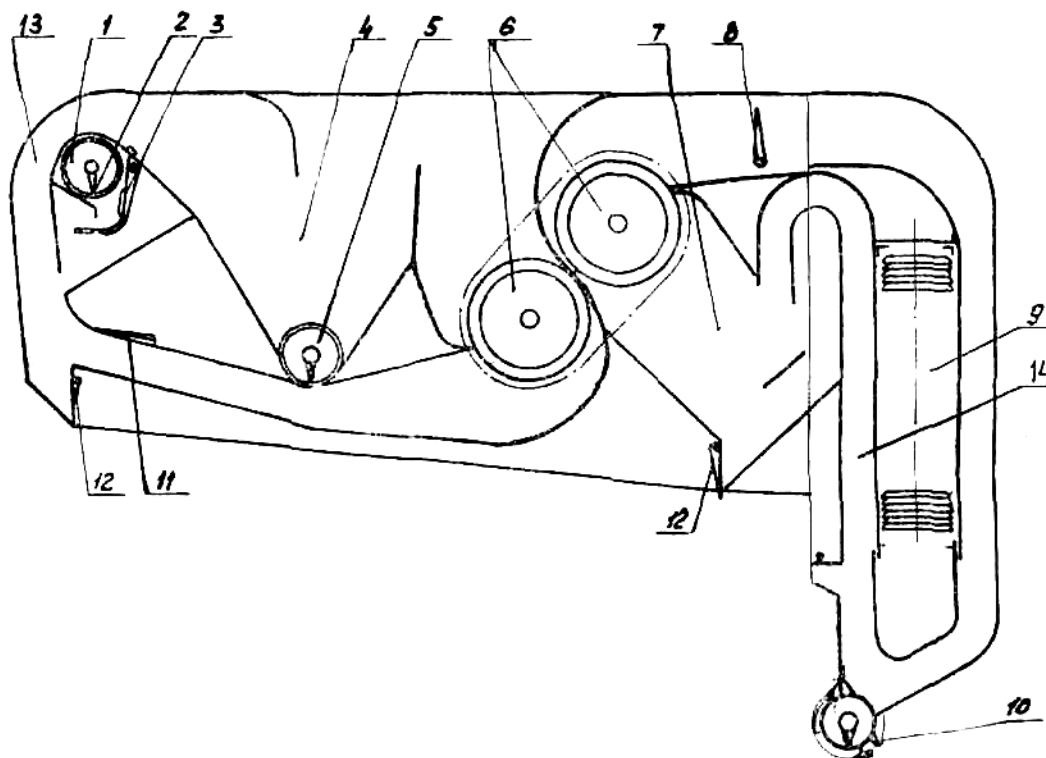
Рис.22.Схема воздушной системы: 1 – шнек; 2 – подвижная перегородка; 3 – клапан-питатель; 4 – отстойная (осадочная) камера 1-ой аспирации; 5 – шнек отходов; 6 – роторы вентилятора; 7 – отстойная (осадочная) камера 2-ой аспирации; 8 – заслонка 2 – ой аспирации; 9 – фильтр; 10 – шнек очищенного зерна; 11 – заслонка 1-ой аспирации; 12 – клапаны; 13 – рабочий канал 1 –ой аспирации; 14 – рабочий канал 2-ой аспирации.
