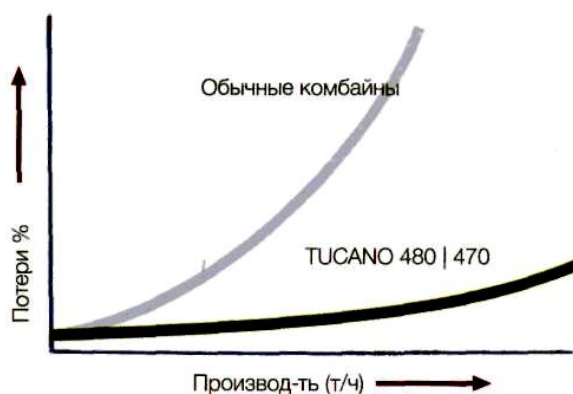
Рис.13. Зависимость потерь зерна от подачи хлебной массы комбайнов классической (обычной) и смешанной (Tucano 480/470) МСС
