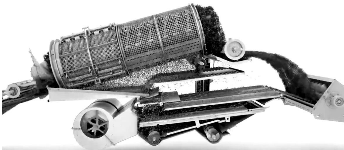
Рис.11. Стоп-кадр технологического процесса работы зерноуборочного комбайна Torum
