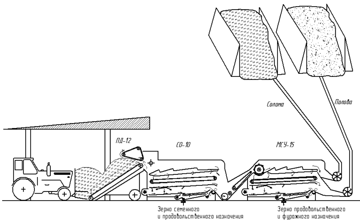
Рис. 3: Схема технологического процесса работы стационарной линии
