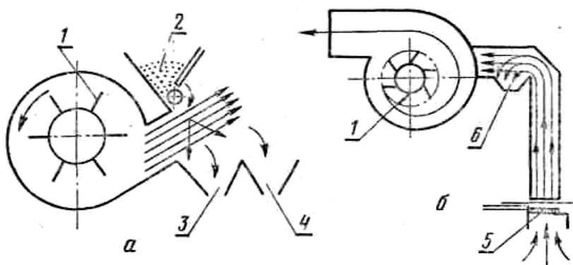
Рис.15. Схемы разделения частиц по парусности: а – в нагнетательном воздушном потоке; б – во всасывающем воздушном потоке; 1 – вентилятор; 2 – бункер (питательный ковш); 3 и 4 – лотки; 5 – сетка; 6 – камера
