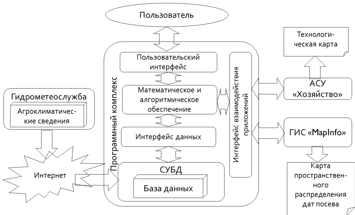
Рисунок 1.14 – Схема функционирования программного комплекса прогнозирования сроков посева
