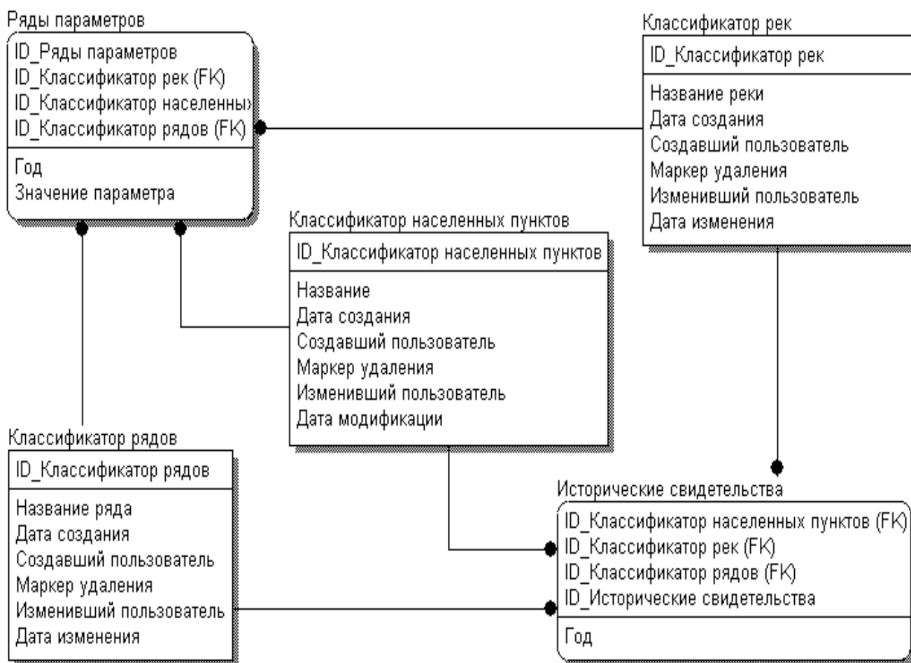
Рисунок 1.20 – Модель базы данных программного комплекса моделирования влияния природных и техногенных событий на планирование
