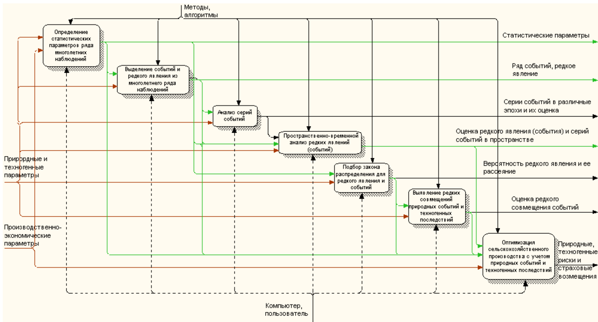
Рисунок 1.19 – Декомпозиция функциональной модели программного комплекса моделирования влияния природных и техногенных событий на планирование
