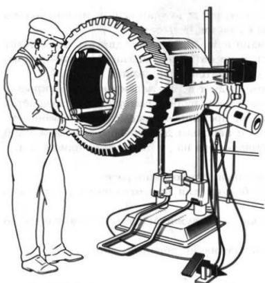
Рисунок 3.12 – Применение пневматического спредера для осмотра шин
