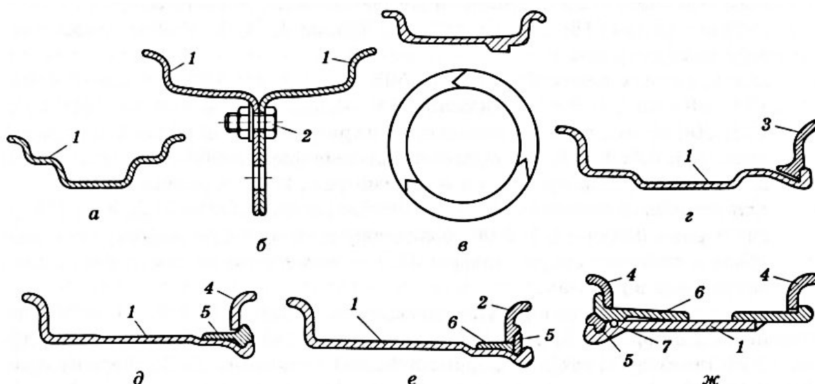
Рисунок 1.8. Основные типы ободьев колес:
