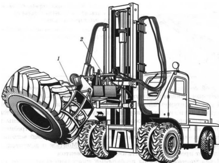
Рисунок 3.1. Приспособление на базе автопогрузчика для снятия сверхкрупногабаритных колес карьерных самосвалов:
