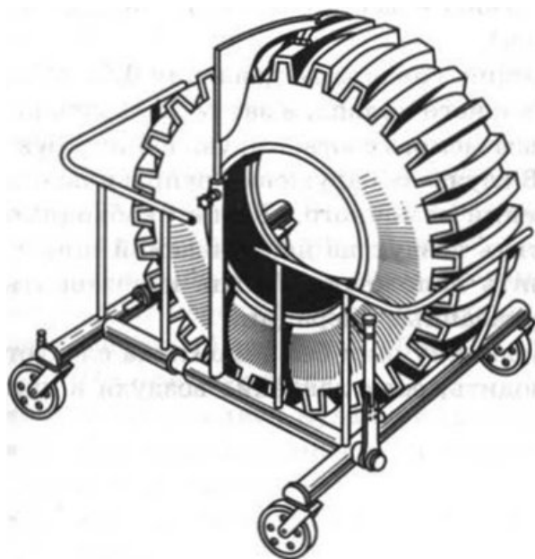
Рисунок 3.2. Универсальная тележка для снятия и транспортировки крупногабаритных колёс
