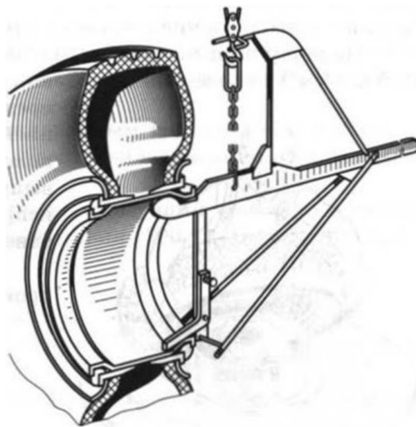
Рисунок 3.3. Приспособление для снятия и установки крупногабаритных колёс
