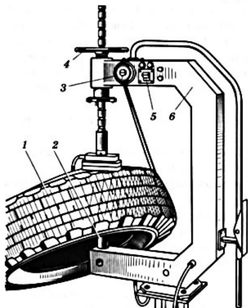
Рисунок 3.18 – Применение вулканизатора для ремонта шин:
