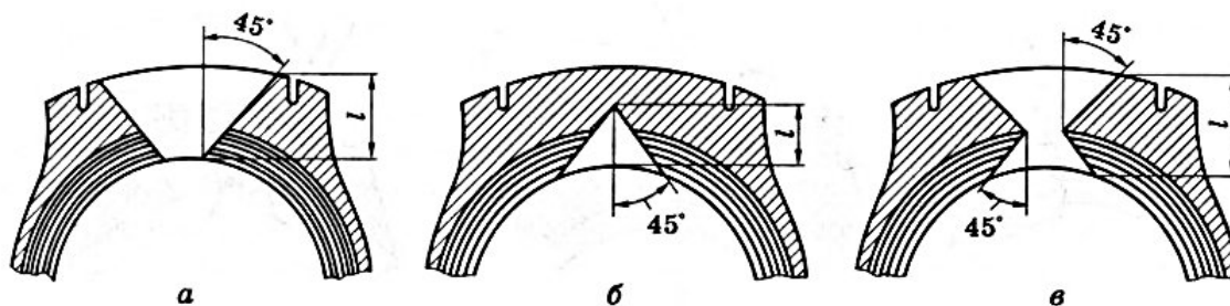
Рисунок 3.13. Способы вырезания поврежденных участков шины: а - «наружный конус»; б - «внутренний конус»; в - «встречный конус»; l - глубина повреждения
