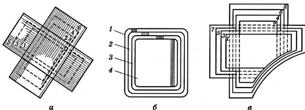
Рисунок 3.15 – Схема расположения слоев пластырей:
