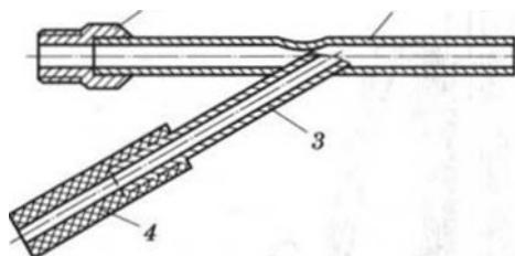
Рисунок 3.4. Инжекторное приспособление для ускорения выпуска воздуха из крупногабаритных шин:
