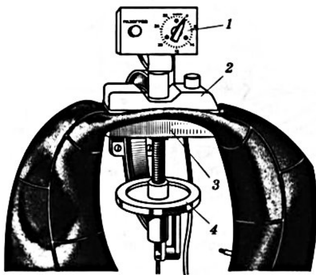
Рисунок 3.10 – Применение вулканизатора при ремонте камеры:
