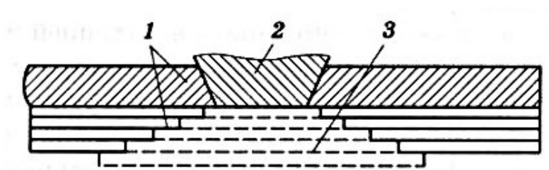
Рисунок 3.16 – Заделка повреждения в случае вырезания участка способом «в рамку»: 1 – прослоечная резина; 2 – протекторная резина; 3 – слой корда
