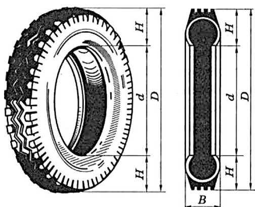
Рисунок 1.4 - Обозначение размеров шин:
