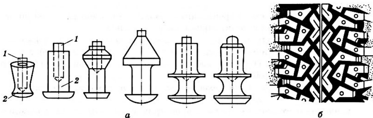
Рисунок 2.1. Шипы противоскольжения (а) и фрагмент шины с шипами (б): 1 - стержень-вставка шипа; 2 - корпус шипа
