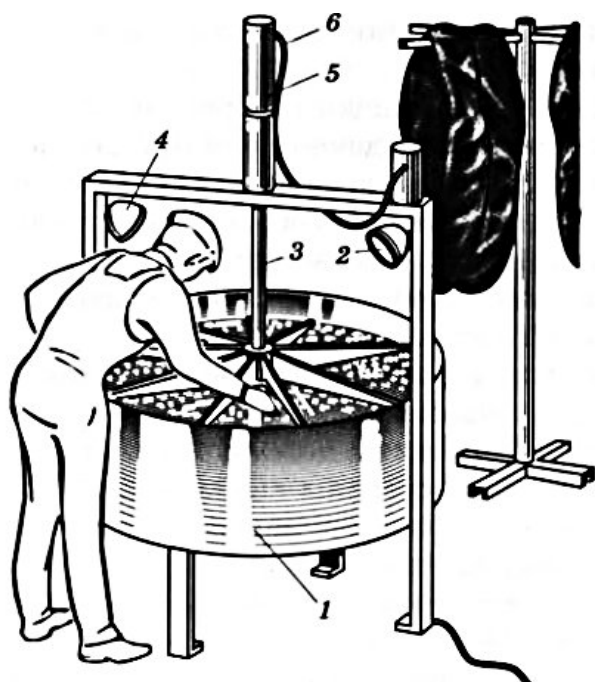
Рисунок 3.11 - Применение ванны для проверки герметичности камер: 1 - ванна; 2, 4 - фонари освещения; 3 - шток утопителя камеры; 5 - пнев- моцилиндр; 6 - шланг подвода сжатого воздуха
