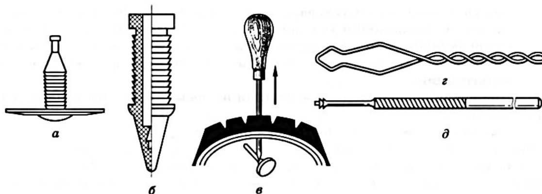
Рисунок 3.19 - Приспособления для ремонта покрышек:
