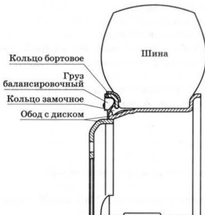
Рисунок 1.6 – Дисковое колесо
