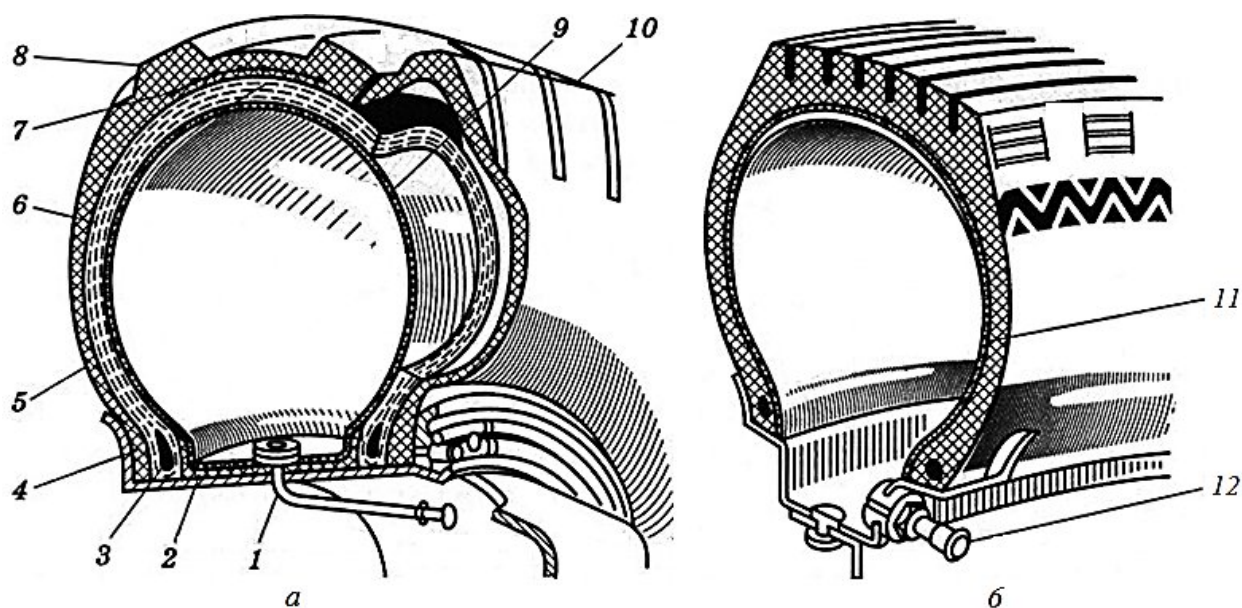
Рисунок 1.2 - Камерная (а) и бескамерная (б) шины:
