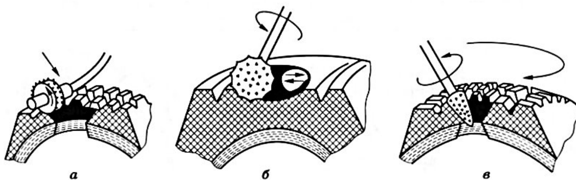
Рисунок 3.14 – Способы шероховки поврежденных мест при ремонте шин:
