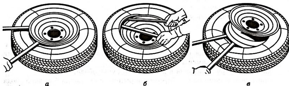
Рисунок 3.8 - Демонтаж шины легкового автомобиля:
