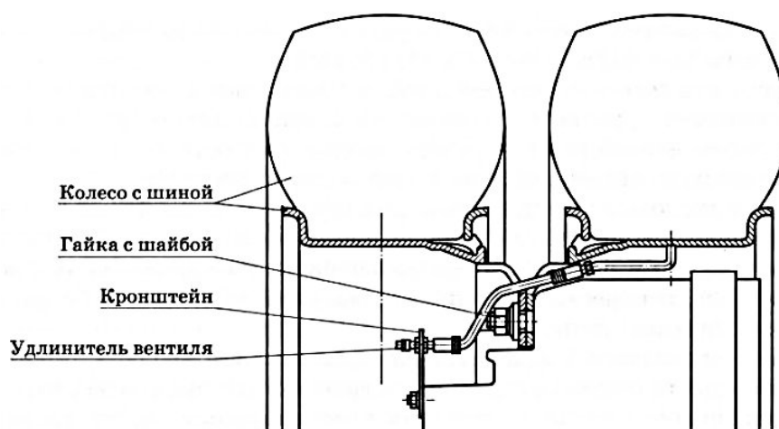
Рисунок 1.7 - Дисковое сдвоенное колесо
