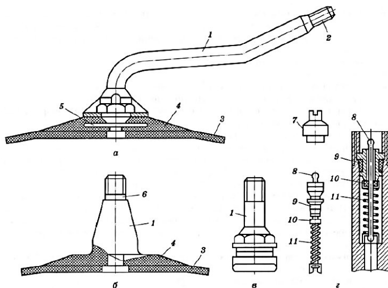
Рисунок 1.5 - Вентили
