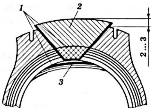
Рисунок 3.17 – Заделка сквозного повреждения в случае вырезания способом «наружный конус»:
