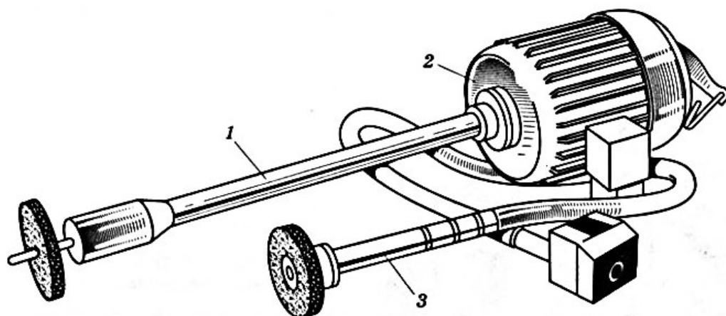
Рисунок 3.9 – Шероховальный станок с гибким приводом и сменными валами: 1 – жесткий вал с цилиндрической проволочной щеткой; 2 – электродвигатель; 3 – гибкий вал
