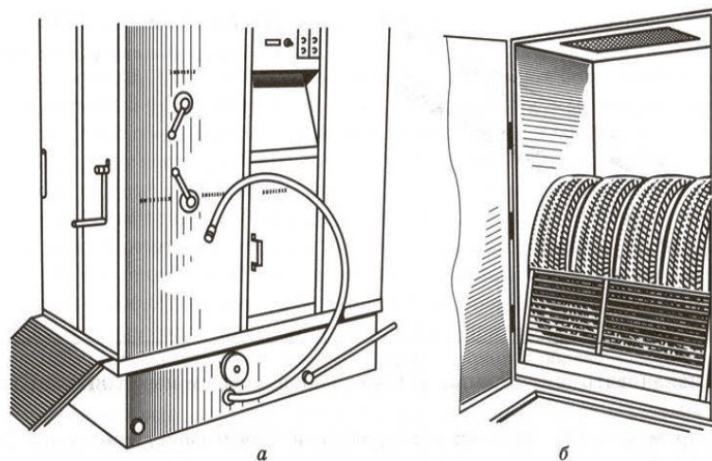
Рисунок 3.6 – Машина для мойки колес (а) и сушильная камера (б)
