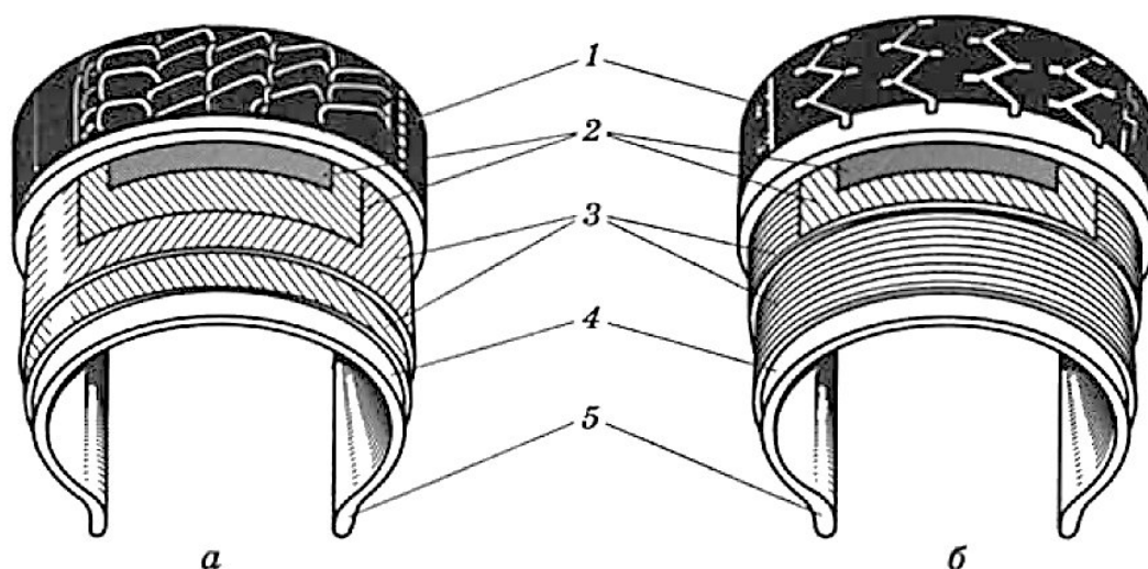
Рисунок 1.3 - Покрышки диагональной (а) и радиальной (б) конструкции (разрез): 1 - протектор; 2 - слой брекера; 3 - слой каркаса; 4 - резиновая прослойка каркаса; 5 - бортовая часть
