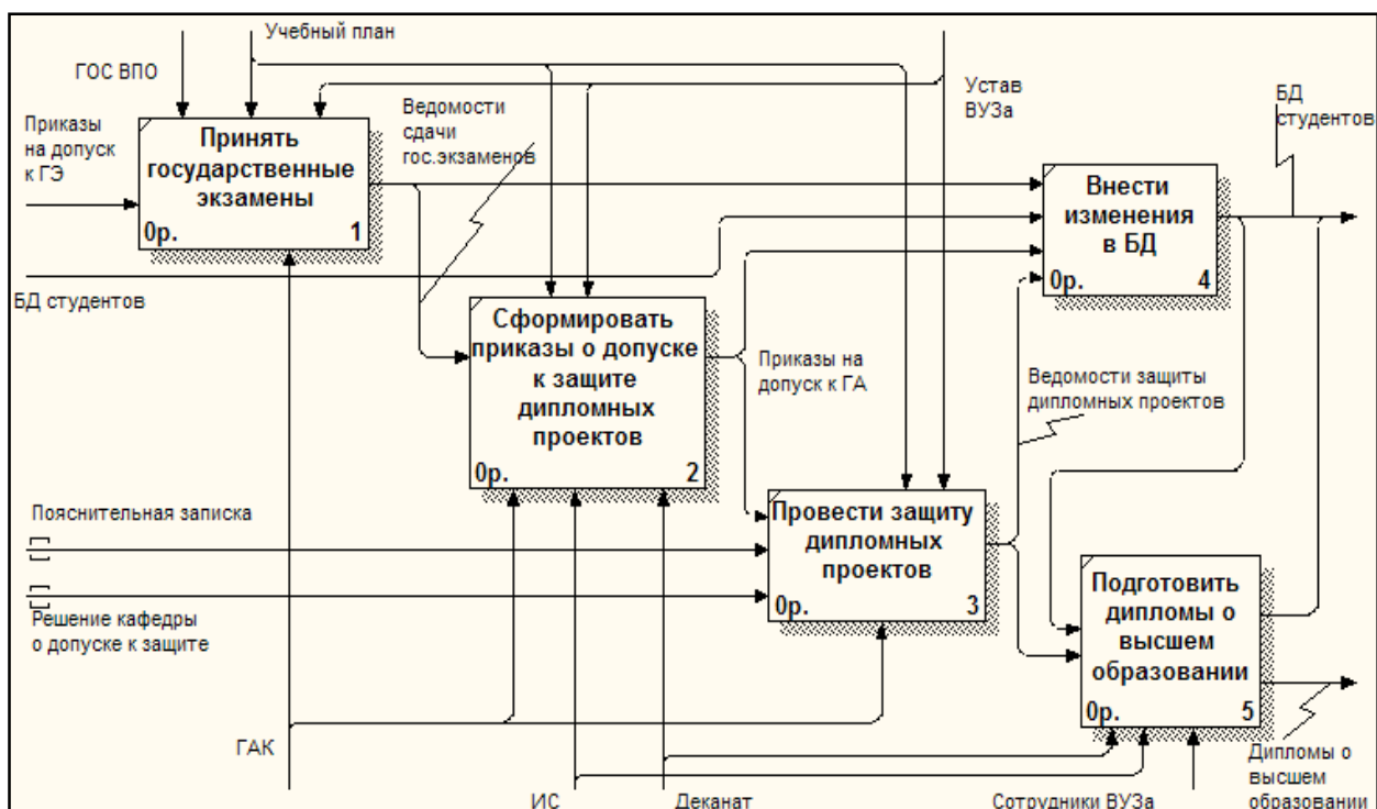
Рисунок 19 – Диаграмма декомпозиции процесса «Выпустить студентов»
