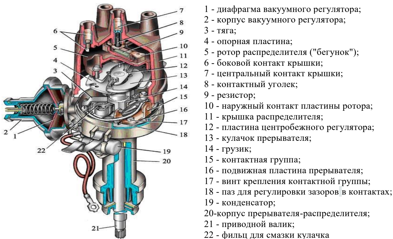
Рисунок 11.3 – Прерыватель-распределитель зажигания
