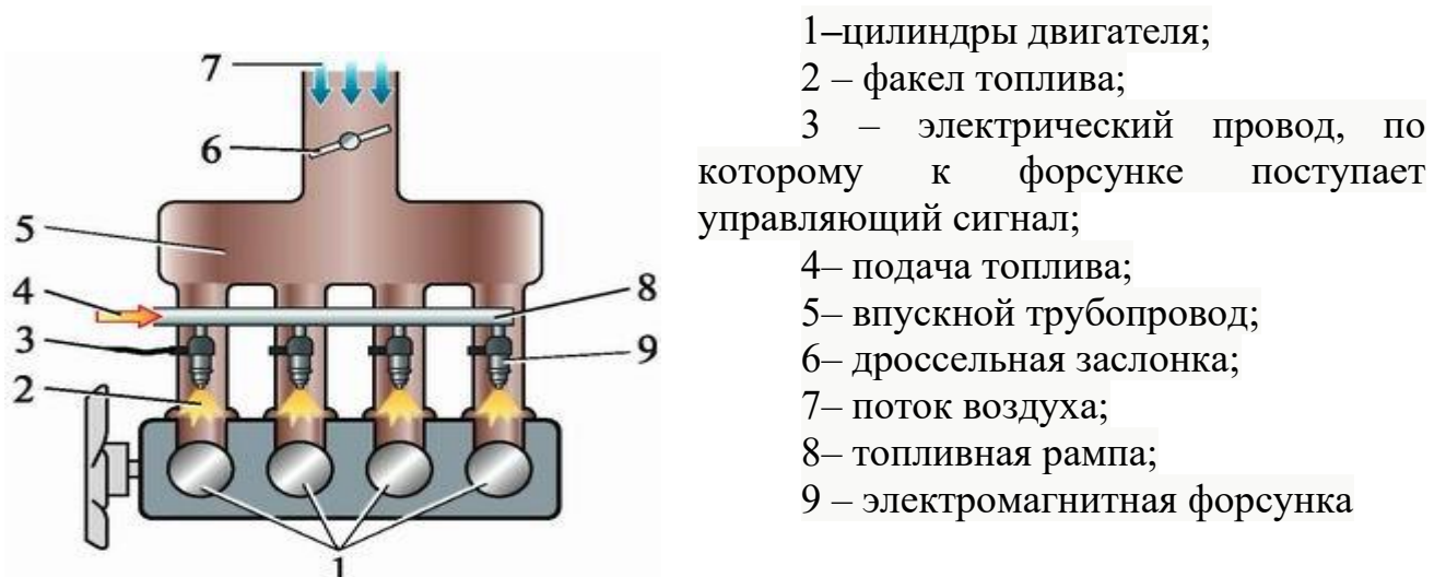
Рисунок 8.2 – Система центрального (моновпрыска, точечного впрыска) впрыска топлива
