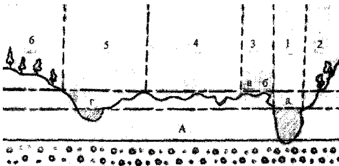
Рис. 2. Профиль через пойму реки. 1 – русло реки ; 2 – надпойменная ераса ; 3 – прирусловая пойма : а – бичевник, б – прирусловой вал; в – прирусловая пойма; 4 – центральная пойма ; 5 – притеррасная пойма : г – притеррасная речка; 6 – вторая надпойменная терраса ; А – уровень грунтовых вод
