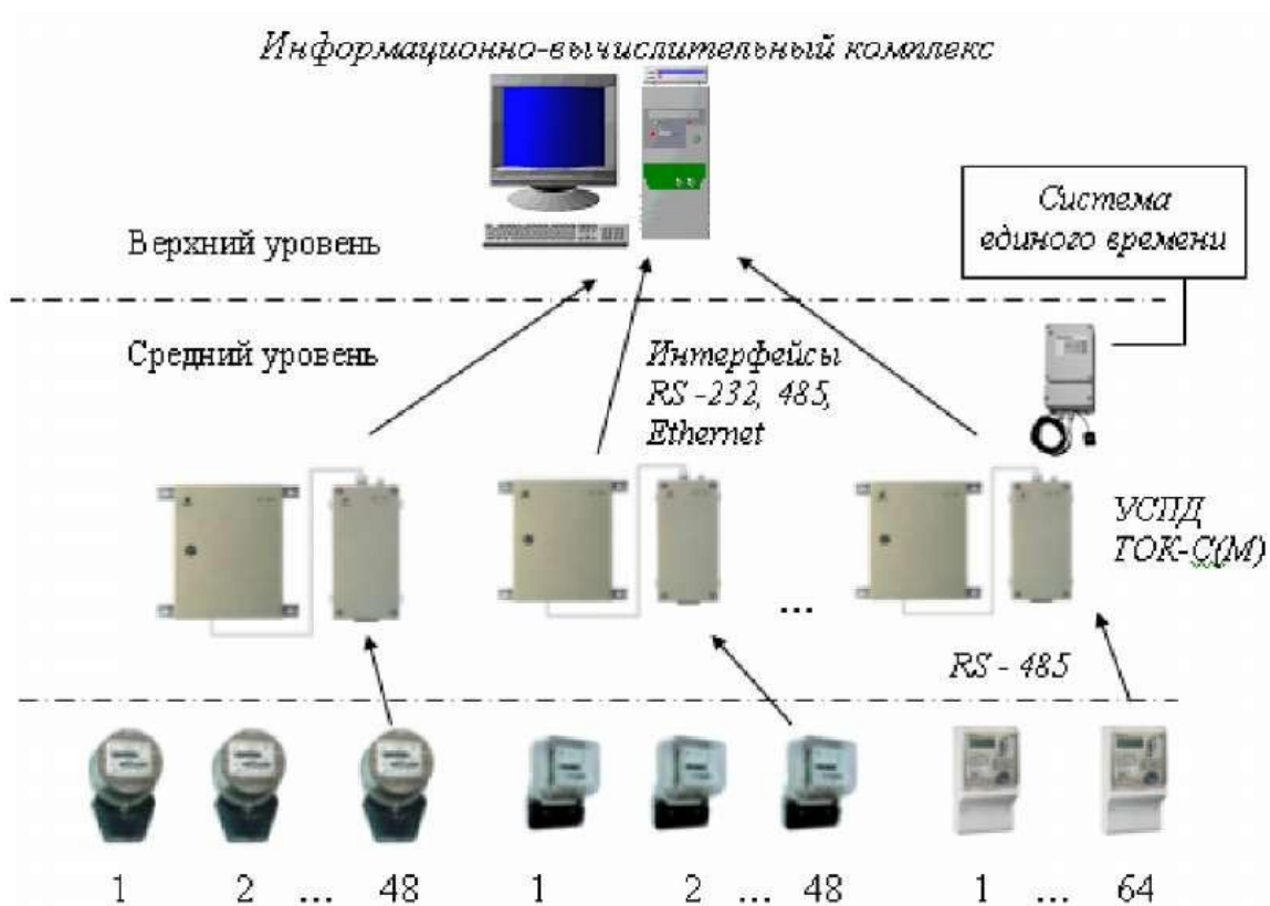
Рисунок 3.1 – Структурная схема локальной АСКУЭ «ТОК-С»
