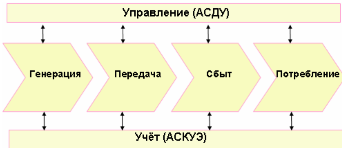
Рисунок 1.3 – Технологический процесс управления электроэнергией
