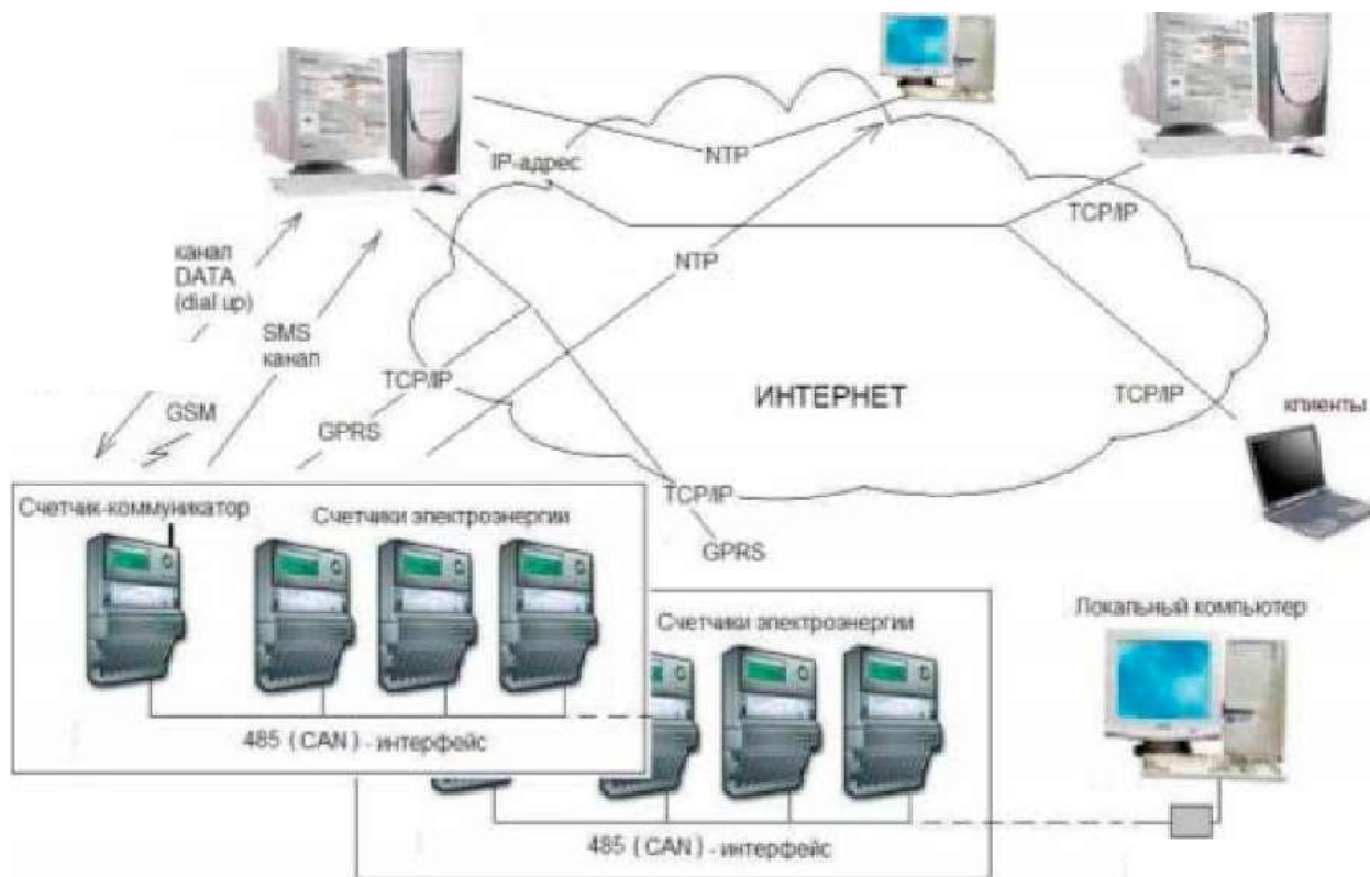
Рисунок 3.4 – Модель информационных процессов системы «ЭКОТЕК»
