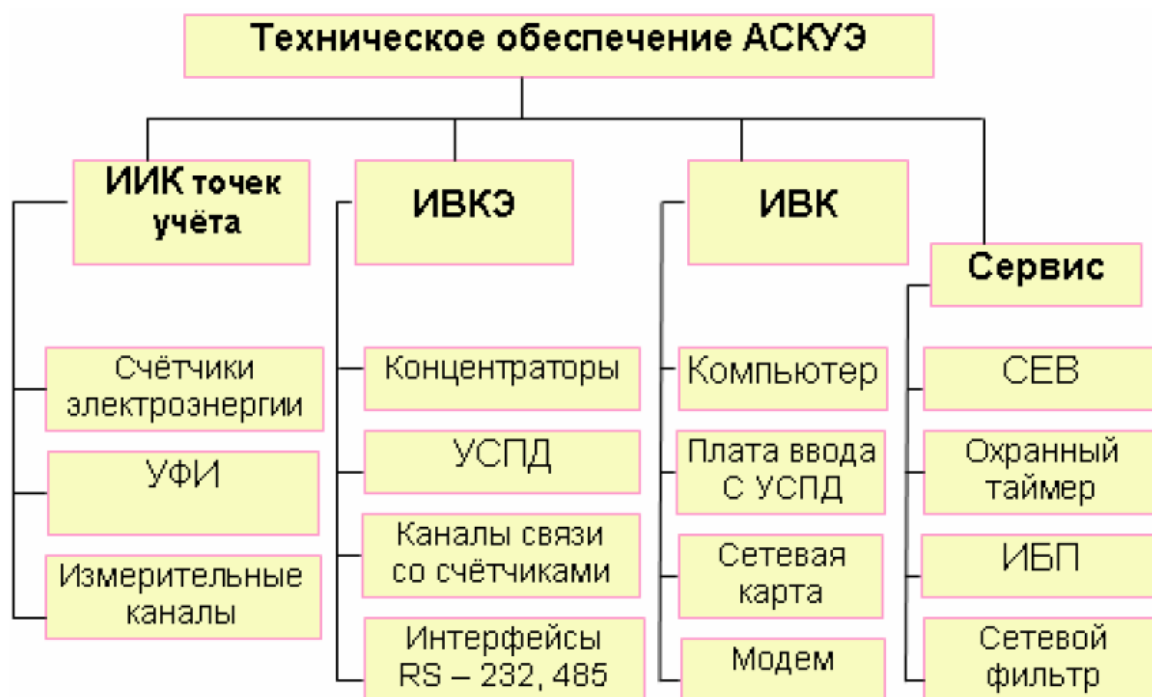
Рисунок 2.2 – Состав технического обеспечения АСКУЭ
