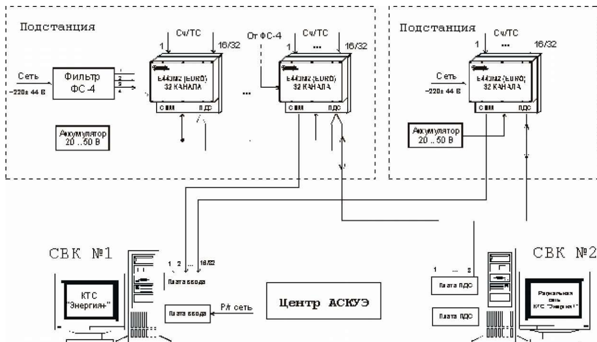
Рисунок 3.2 – Высоконадежная АСКУЭ, построенная на базе КТС «Энергия+»
