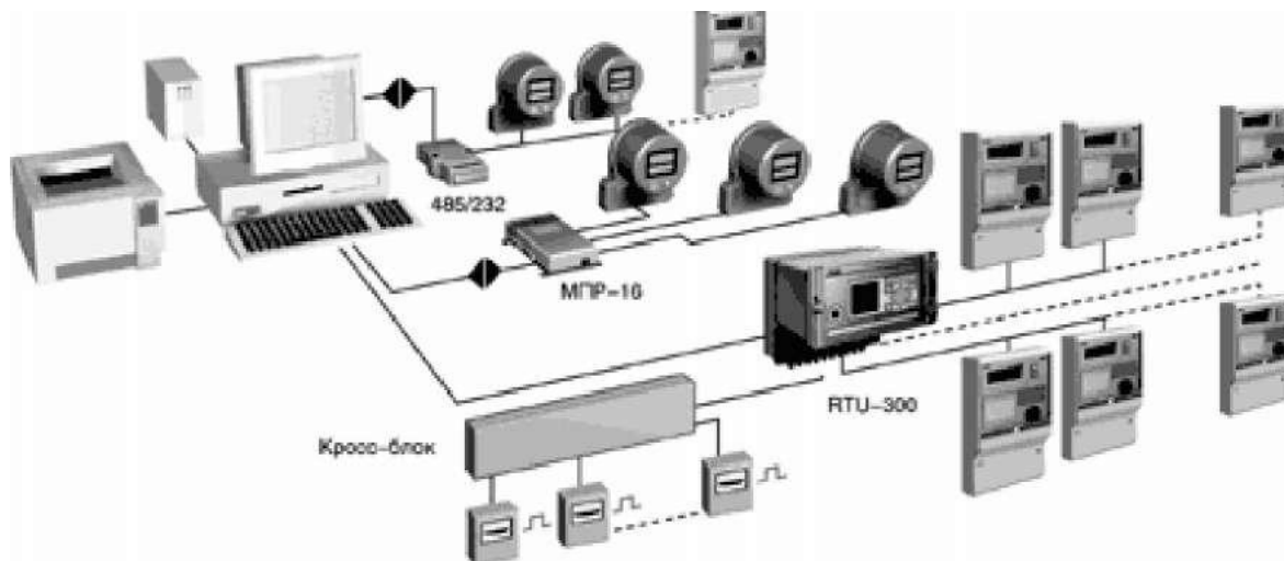
Рисунок 3.3 – Вариант АСКУЭ «АльфаЦЕНТР» с локальной сетью
