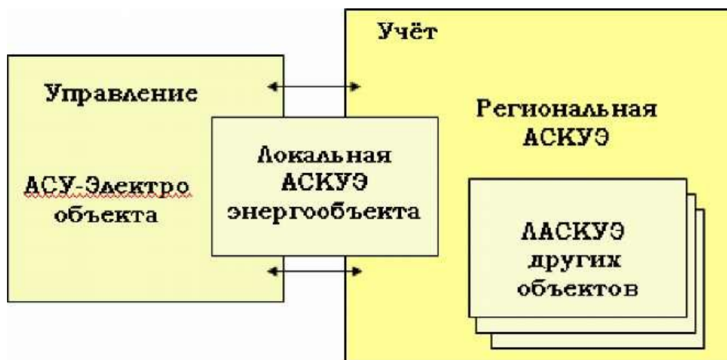
Рисунок 1.4 – Локальная и региональная АСКУЭ
