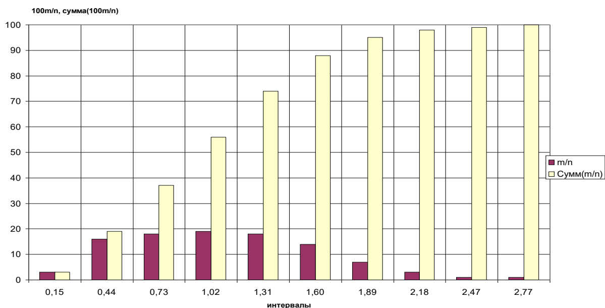
Рисунок 2.6 - Гистограмма и огиба смоделированной связной выборки нормального закона распределения при k=1 , C_v=0,5 , r=0,4 и n=100
