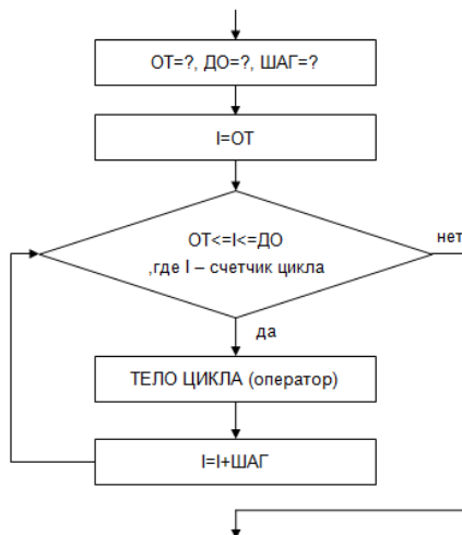
Блок-схема цикла FOR.
