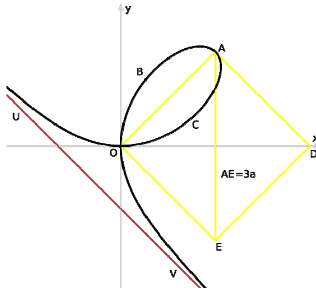
Рис. 11.1. Декартов лист
