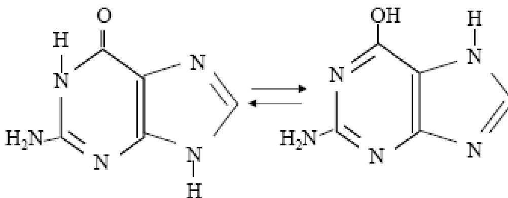
лактимная форма
