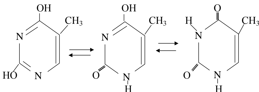
тимин (2,4дигидрокси5метилпиримидин)
