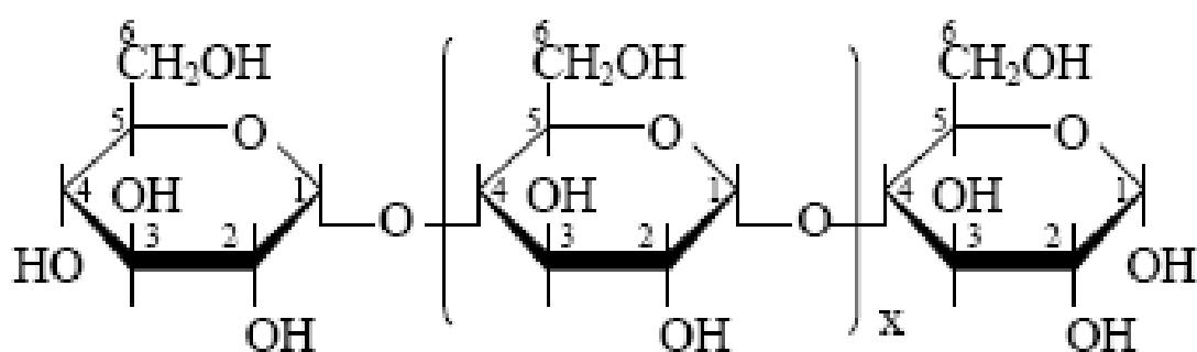
амилоза
