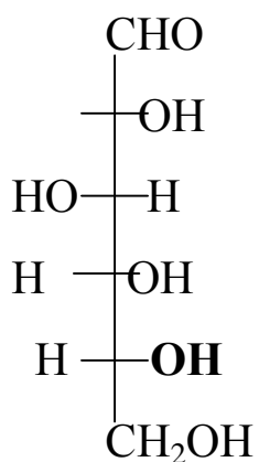
D– глюкоза
