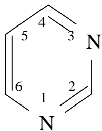
Пиримидин (1,3-диазин)
