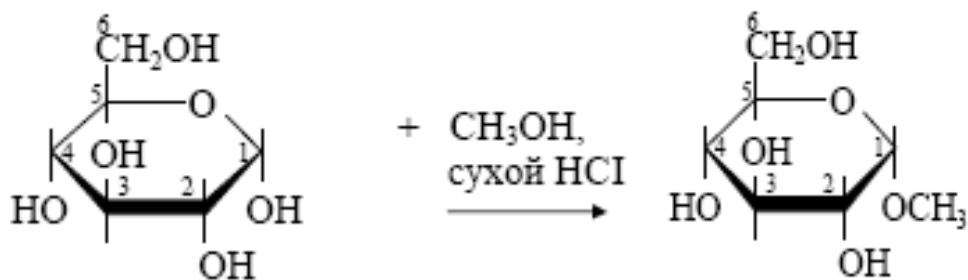
D– глюкопираноза
