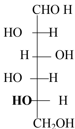
L– глюкоза
