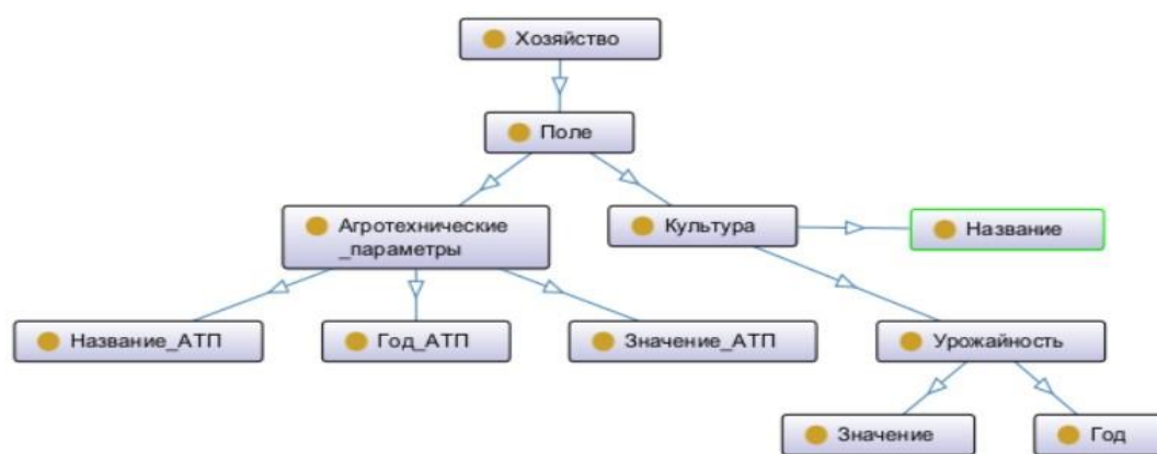
Рисунок 1 – Описание класса «Хозяйство»
